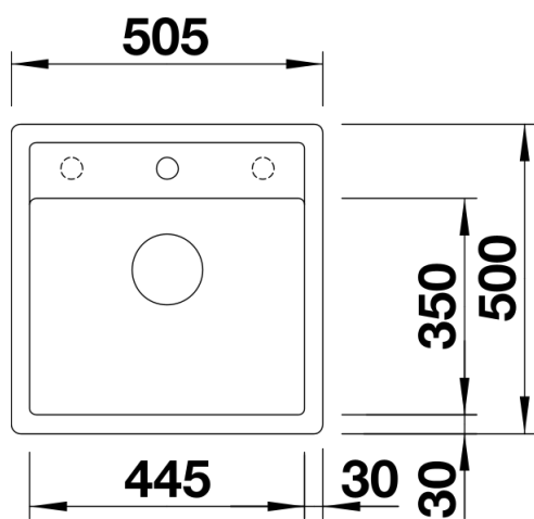
Aufsicht
